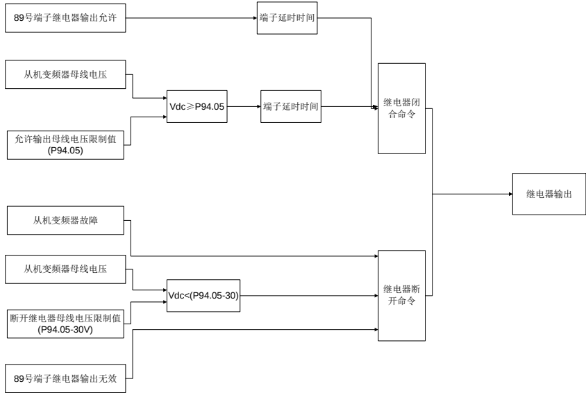
图 5-23 继电器输出控制逻辑
