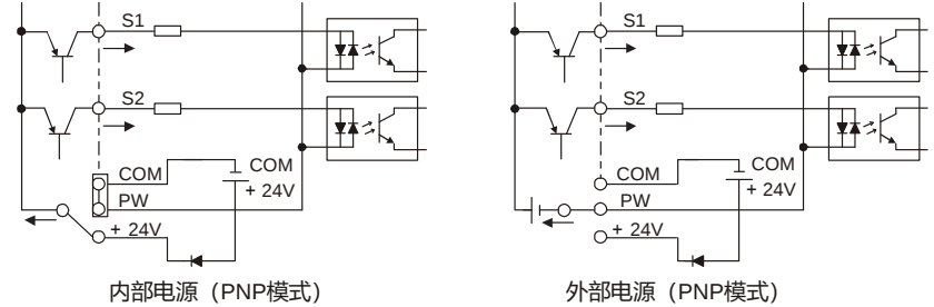
图 4-17 PNP 模式
