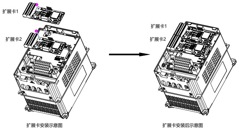
图 A-2 1R5G/2R2P 机型
