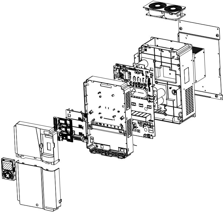
图 C-3 变频器结构
