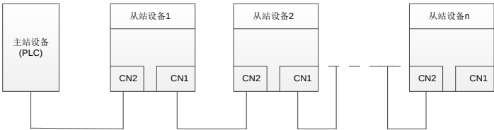
图 A-8 线型网络拓扑电气连接
