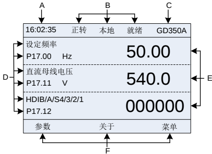
图 5-2 液晶显示器主界面
