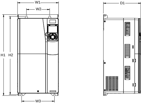
图 C-5 055G/075P~075G/090P 壁挂安装
