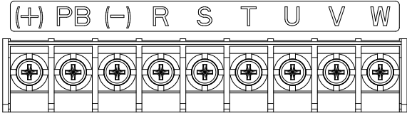
图 4-8 7R5G/011P（含）以下主回路端子
