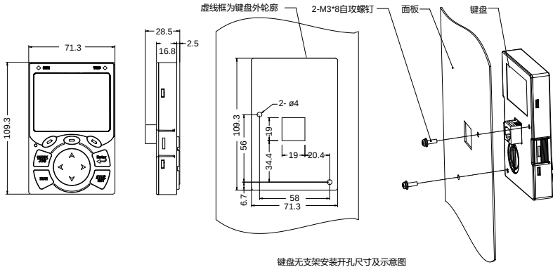
图 C-1 键盘结构
