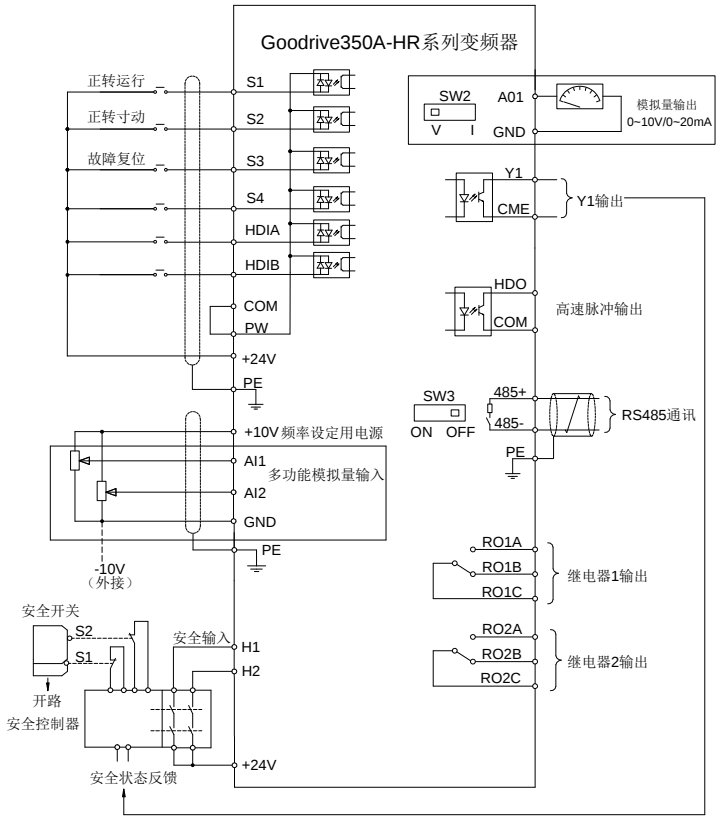
图 4-14 控制回路接线
