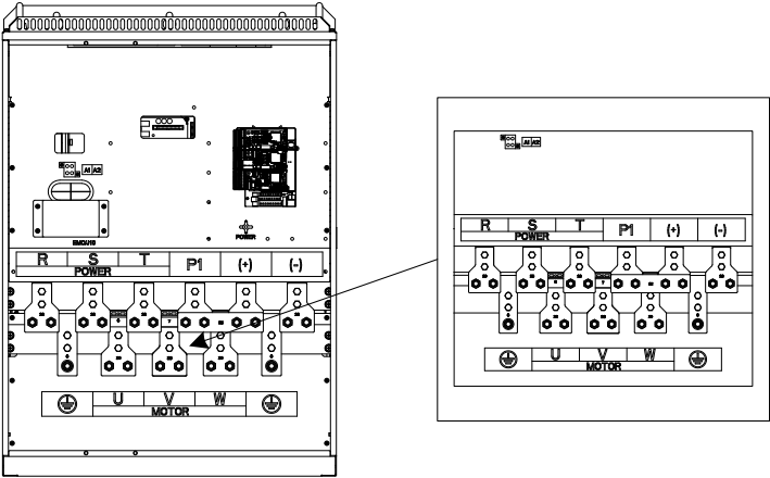
图 4-11 220G/250P~315G/355P 主回路端子
