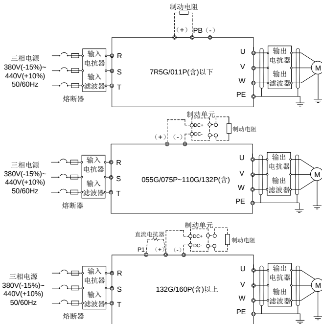
图 4-7 主回路接线
