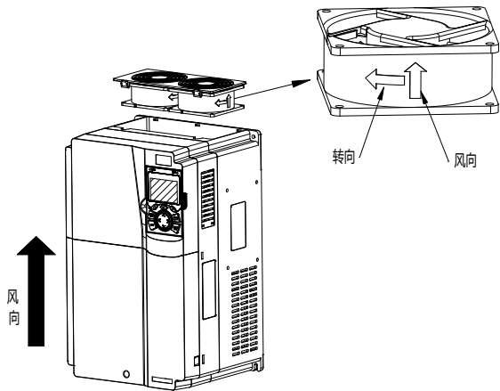
图 9-1 7R5G/011P（含）以上机器风扇维护
