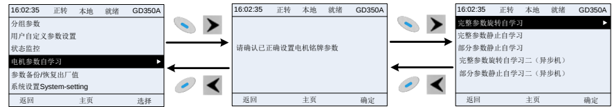
图 5-18 参数自学习操作
