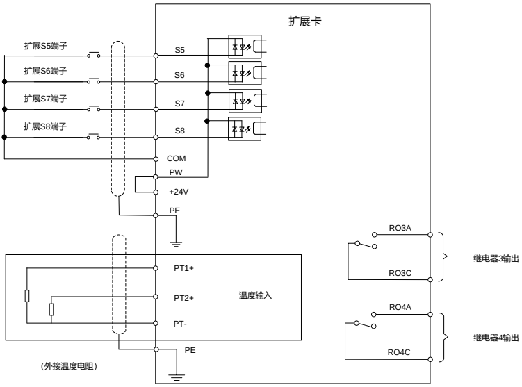
图 A-6 IO 扩展卡 2 控制回路接线
