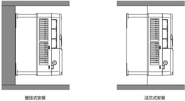
图 4-2 安装方式
