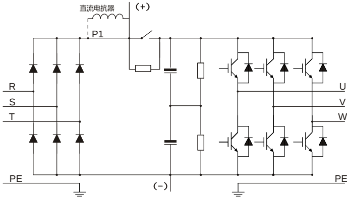
图 3-3 132G/160P~315G/355P 主回路简图
