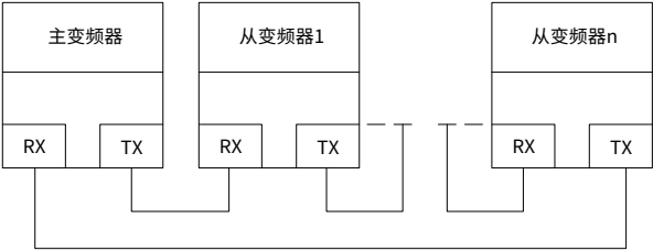
图 A-11 环型网络拓扑电气连接
