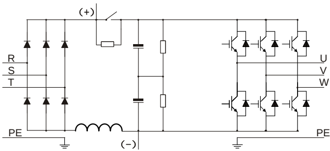
图 3-2 055G/075P~110G/132P 主回路简图
