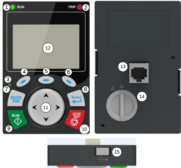
图 5-1 键盘示意图
