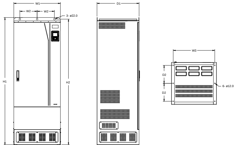
图 C-13 355G/400P~500G 落地安装
