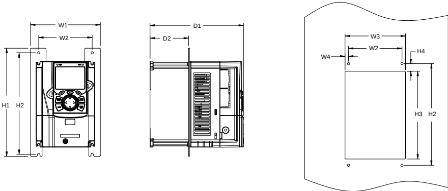
图 C-9 1R5G/2R2P~075G/090P 法兰安装
