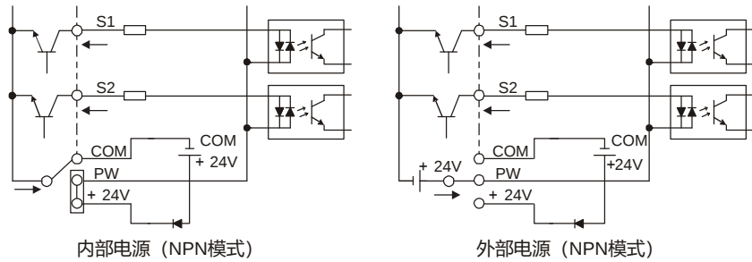
图 4-16 NPN 模式
