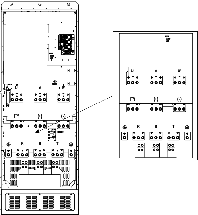
图 4-12 355G/400P~500G 主回路端子
