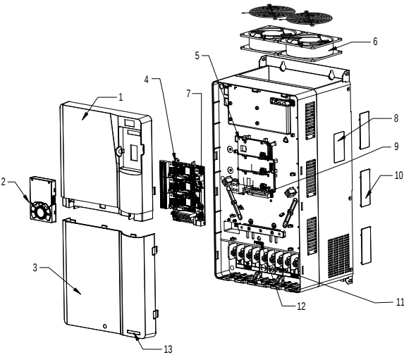
图 3-7 产品结构
