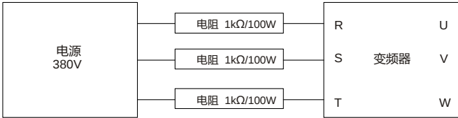
图 9-2 380V 驱动装置充电电路示例
