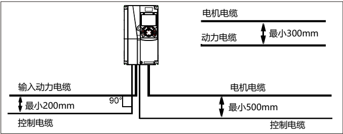
图 D-3 布线距离
