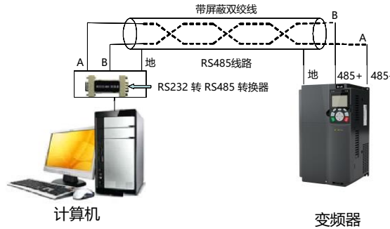
图 10-1 RS485 单机应用时的物理接线
