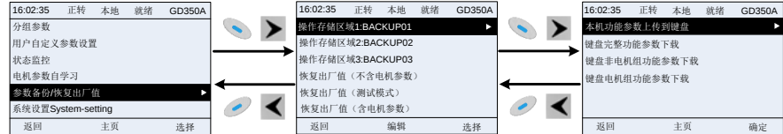
图 5-20 参数备份操作
