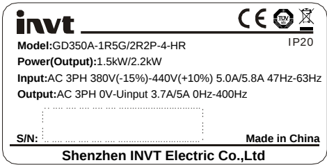
图 3-5 产品铭牌
