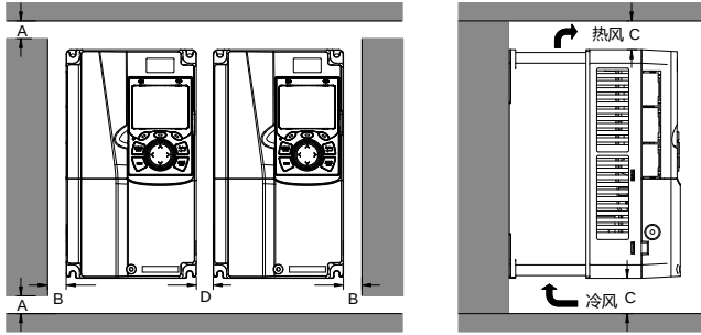
图 4-4 并行安装
