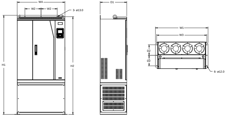
图 C-12 220G/250P~315G/355P 落地安装
