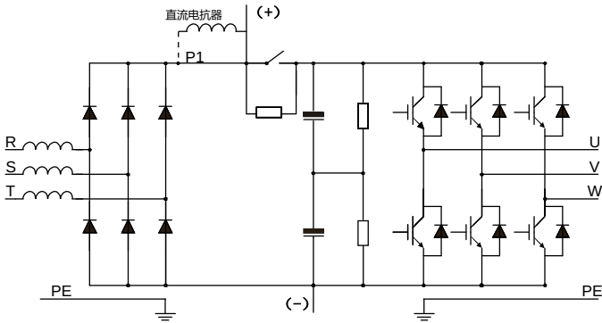
图 3-4 355G/400P 及以上主回路简图
