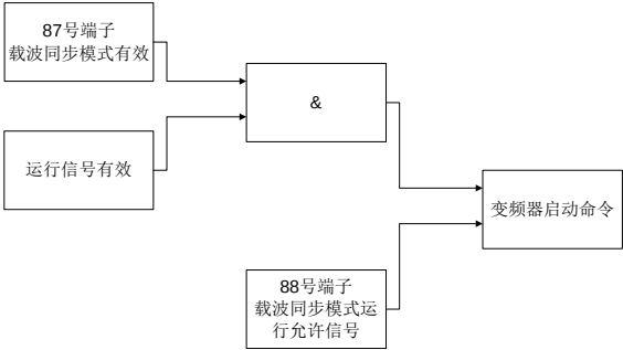
图 5-22 运行命令逻辑
