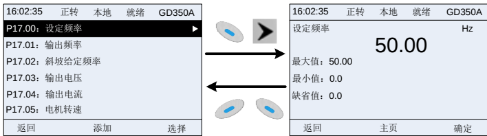
图 5-17 状态监控界面
