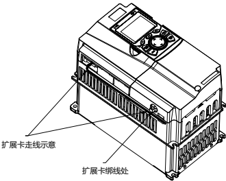
图 A-5 走线方式
