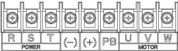
图 4-9 055G/075P~110G/0132P 主回路端子（选配内置制动单元需启用 PB）
