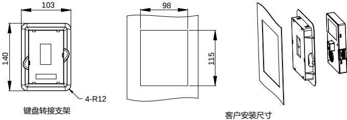
图 C-2 键盘安装架（选配）
