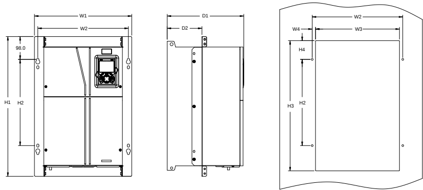
图 C-10 090G/110P~110G/132P 法兰安装
