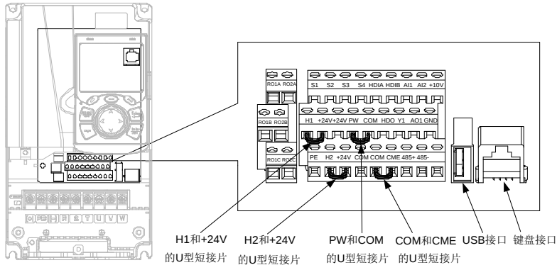
图 4-15 U 型短接位置
