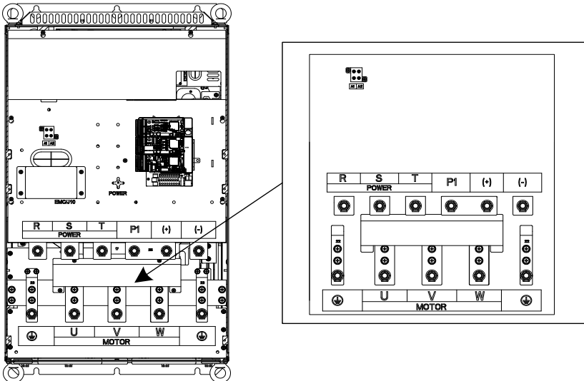
图 4-10 132G/160P~200G/220P 主回路端子
