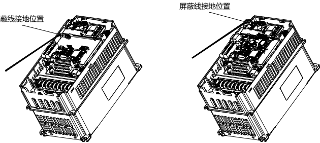
图 A-4 扩展卡地线连接
