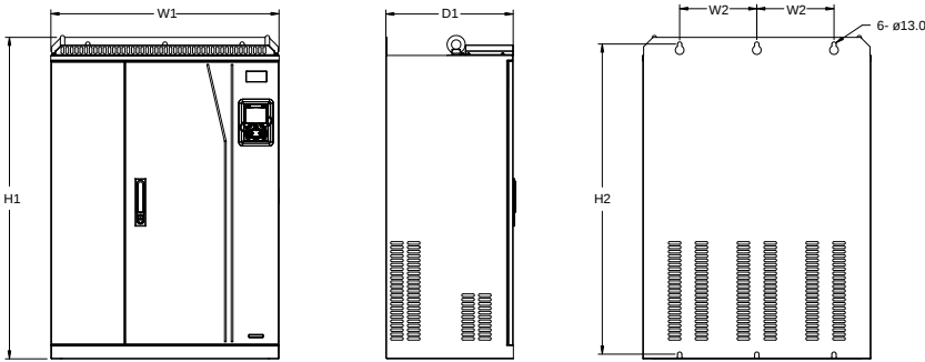
图 C-8 220G/250P~315G/355P 壁挂安装
