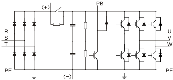
图 3-1 7R5G/011P（含）以下主回路简图
