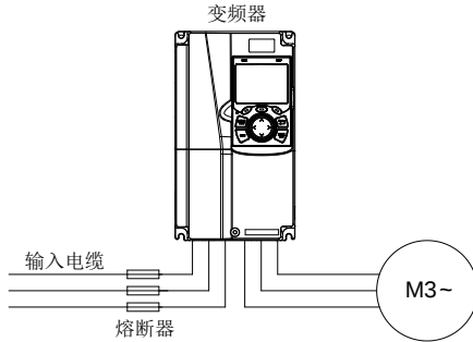
图 4-18 熔断器配置
