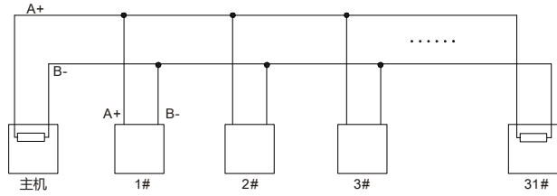
图 10-3 菊花简化接线
