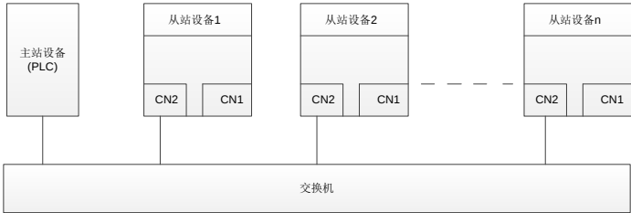
图 A-9 星型网络拓扑电气连接
