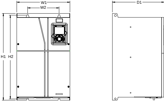
图 C-6 090G/110P~110G/132P 壁挂安装
