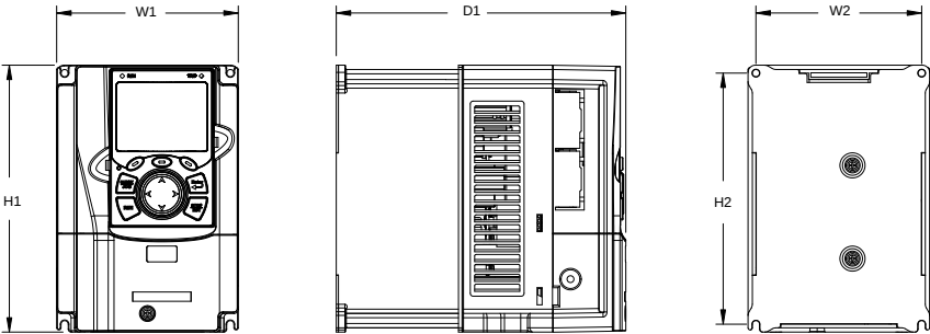
图 C-4 1R5G/2R2P~7R5G/011P 壁挂安装
