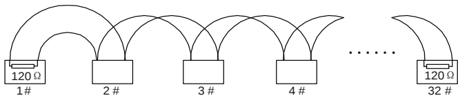
图 11-2 菊花接法现场接线
