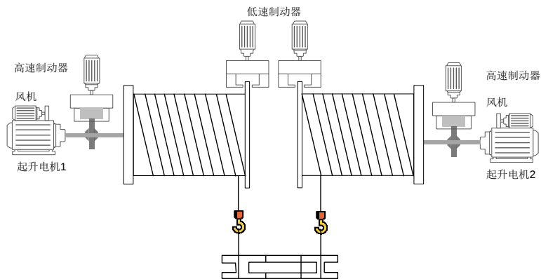
图 5-11 机械结构 2
