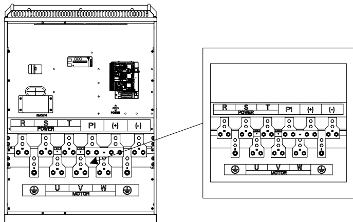
图 4-11 380V 220~315kW 主回路端子
