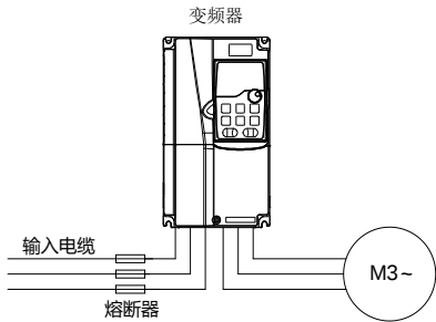
图 4-19 熔断器配置
