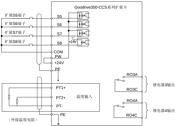
图 4-17 I/O 扩展卡 2 控制回路接线
