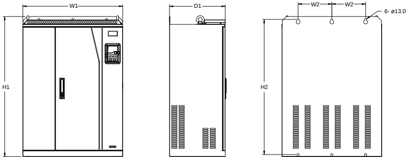
图 C-7 380V 220~315kW 壁挂安装
