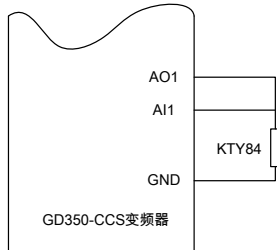
图 5-14 模拟量端口与 KTY84 接线
