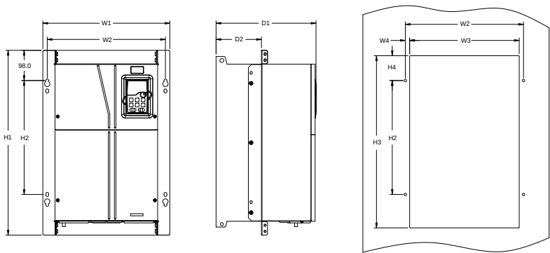
图 C-9 380V 90~110kW 法兰安装
