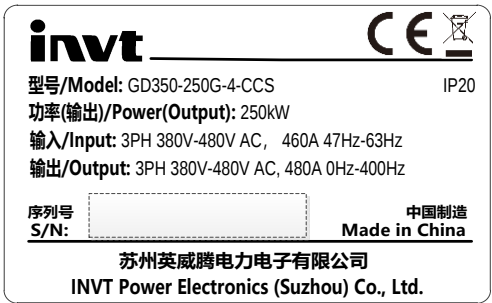
图 3-4 产品铭牌
