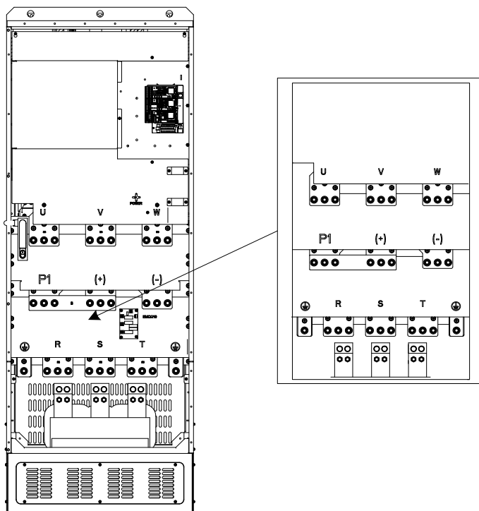
图 4-12 380V 355~500kW 主回路端子
