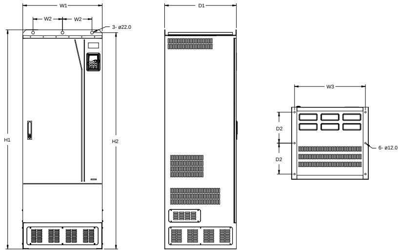
图 C-12 380V 355~500kW 落地安装
