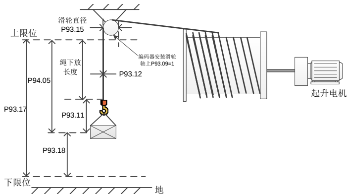
图 5-5 外部测量（HDI）
