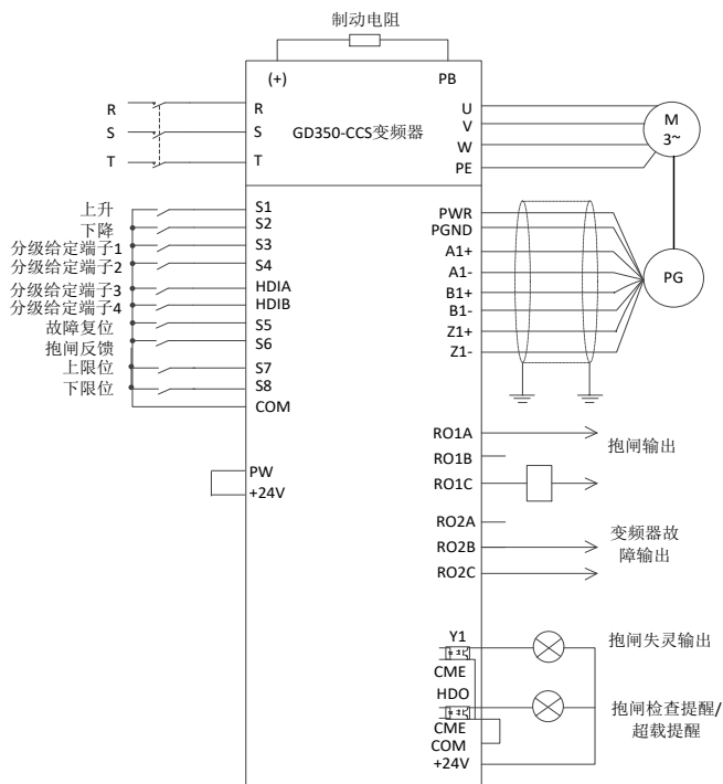
图 5-4 内部测量（电机编码器）接线
