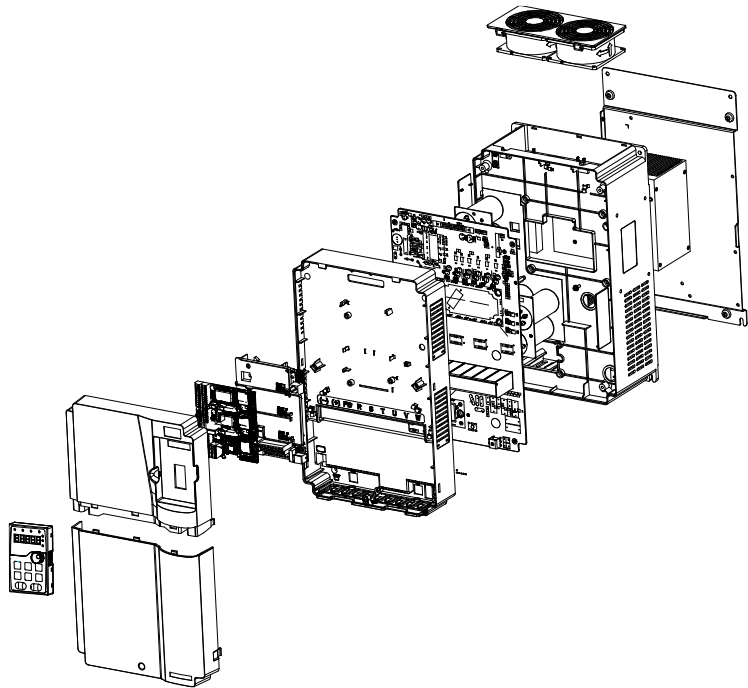
图 C-2 变频器结构
