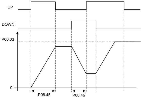
图 5-9 电动电位器调试
