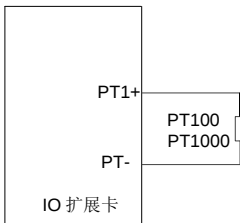
图 5-12 PT100/PT1000 使用扩展卡进行温度测量
