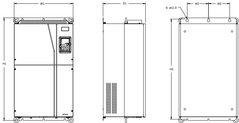
图 C-6 380V 132~200kW 壁挂安装
