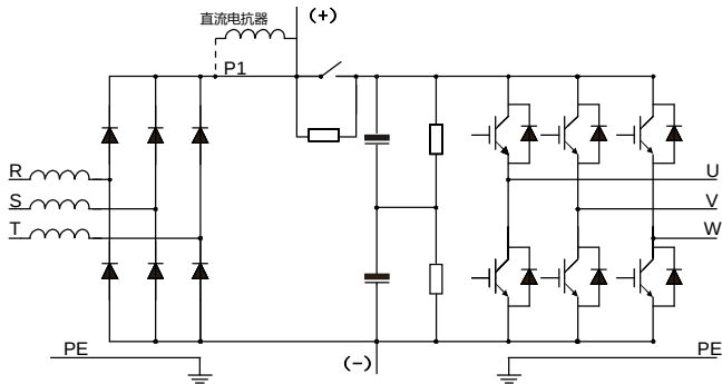
图 3-3 380V 355kW 及以上主回路
