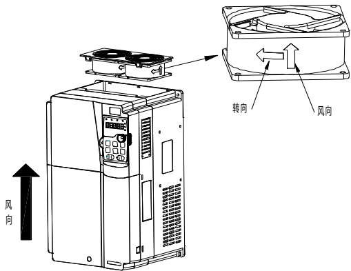
图 10-1 7.5kW 及以上机器风扇维护
