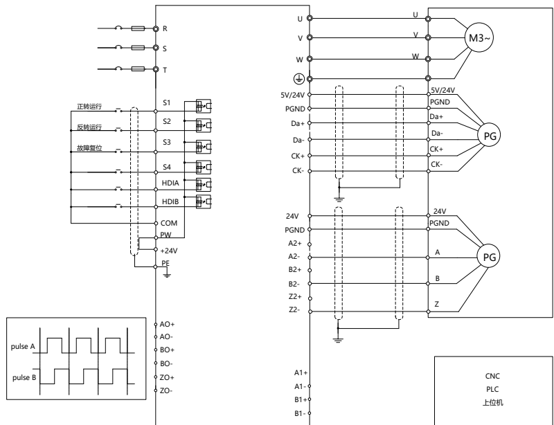
图 A-8 全闭环接 SSI 绝对式编码器和 24V 推挽输出增量式编码器
