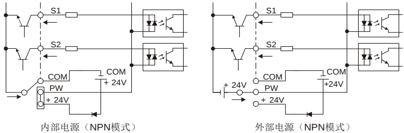
图 4-15 NPN 模式
