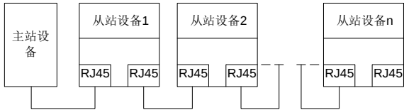
图 A-5 线型网络拓扑电气连接
