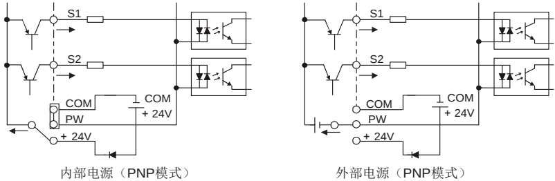
图 4-16 PNP 模式
