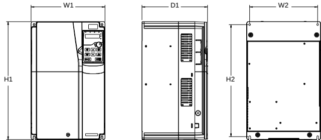
图 C-3 380V 30~37kW 壁挂安装
