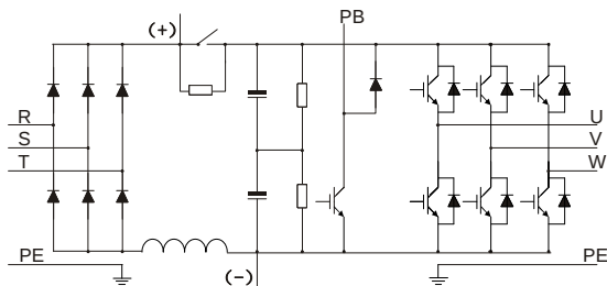
图 3-1 380V 30kW~110kW 主回路
