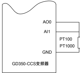
图 5-13 模拟量端口与 PT100/PT1000 接线
