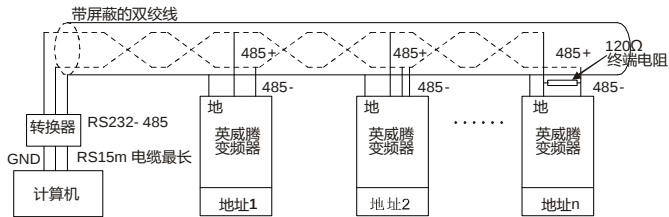
图 11-4 菊花接法运用
