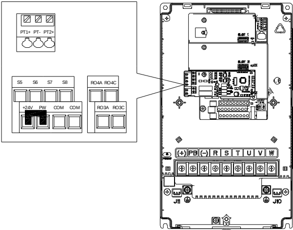
图 4-18 I/O 扩展卡 2 端子排列
