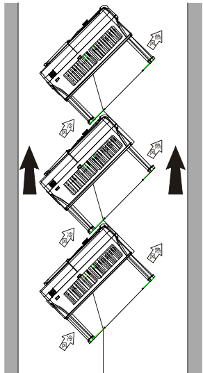
图 4-6 倾斜安装
