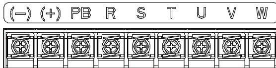
图 4-8 三相 380V 30~37kW 主回路端子
