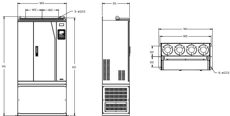
图 C-11 380V 220~315kW 落地安装
