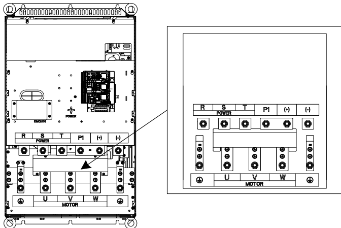
图 4-10 380V 132~200kW 主回路端子
