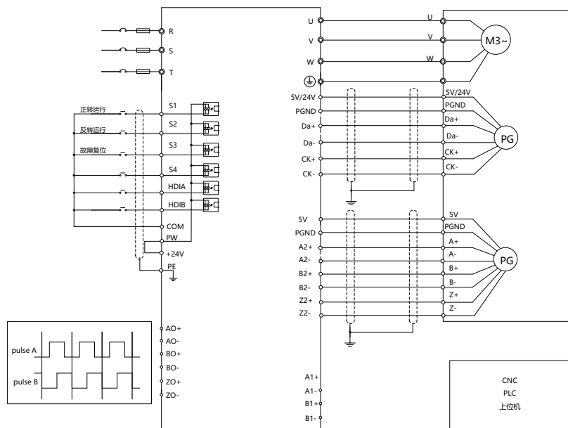
图 A-6 全闭环接 SSI 绝对式编码器和 5V 差分增量式编码器
