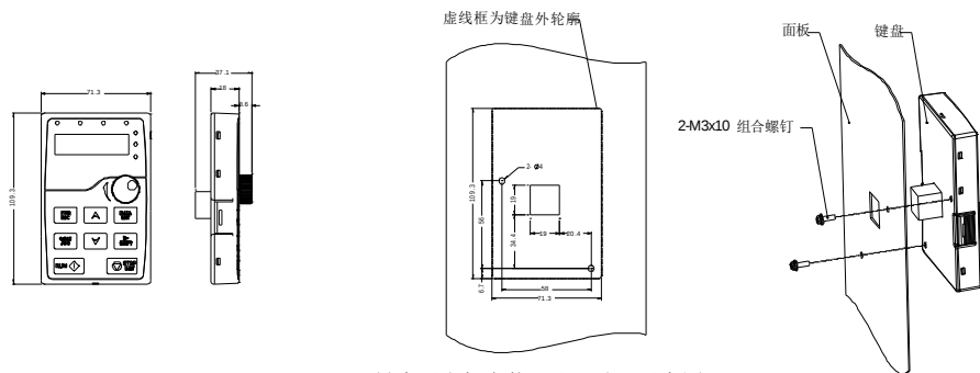
键盘无支架安装开孔尺寸及示意图
