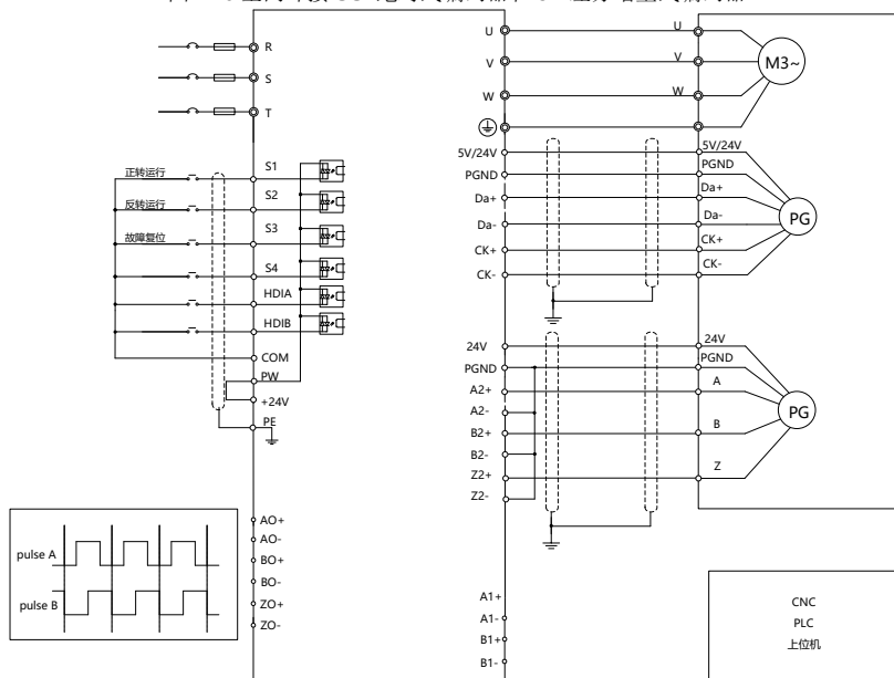
图 A-7 全闭环接 SSI 绝对式编码器和 24V 集电极开路信号增量式编码器
