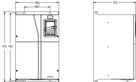
图 C-5 380V 90~110kW 壁挂安装
