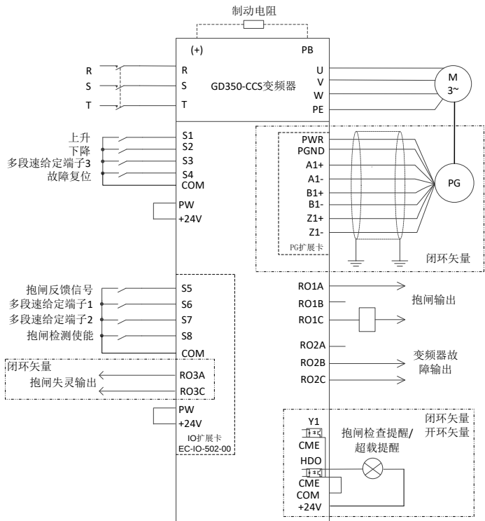
图 5-1 提升应用接线
