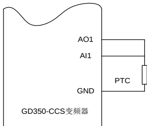
图 5-15 模拟量端口与 PTC 接线
