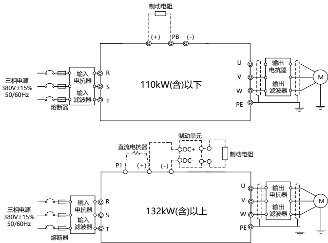
图 4-7 AC 3PH 380V-480V 主回路接线
