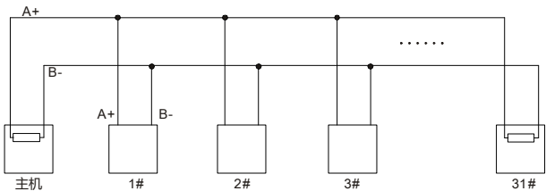
图 11-3 菊花简化接线
