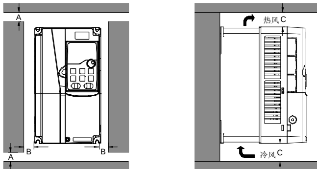
图 4-3 单台安装
