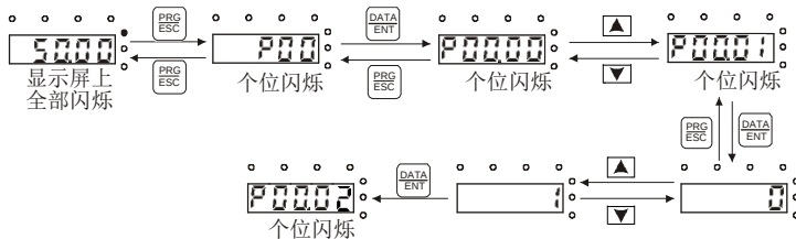
图 6-3 修改参数
