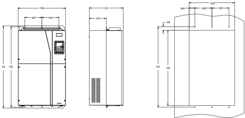
图 C-10 380V 132~200kW 法兰安装
