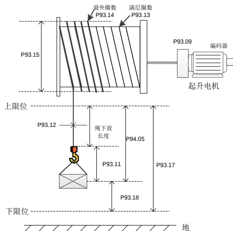
图 5-3 内部测量（电机编码器）：未使用滑轮组
