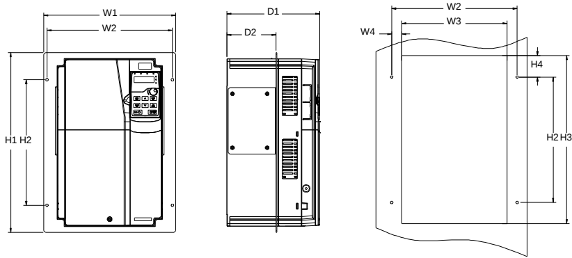
图 C-8 380V 30~75kW 法兰安装
