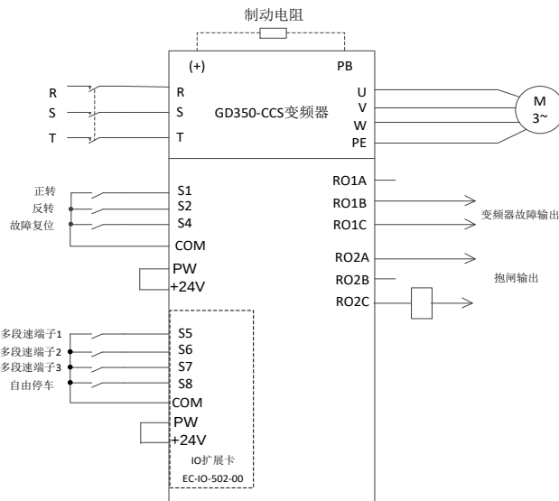
图 5-7 平移应用调试
