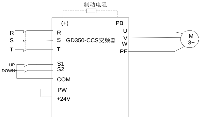
图 5-8 电动电位器调试接线
