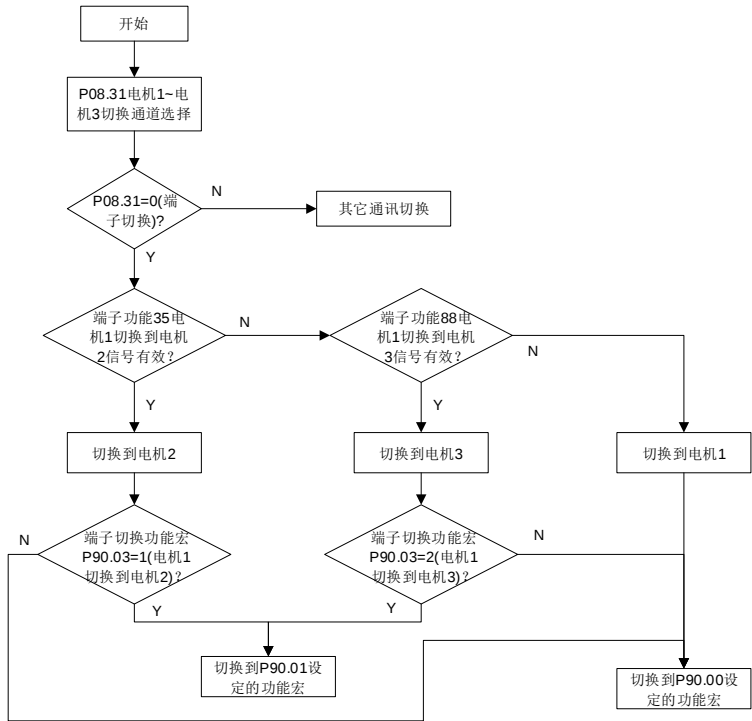
5.5.4 多组电机端子切换和应用宏切换流程图
