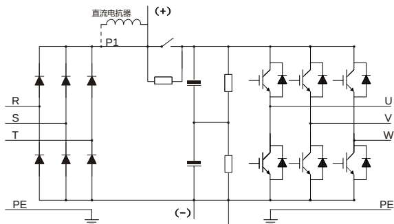
图 3-2 380V 132kW~315kW 主回路
