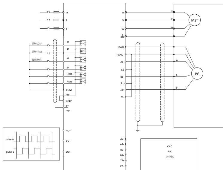
与推挽型编码器配套使用时的外部接线图
