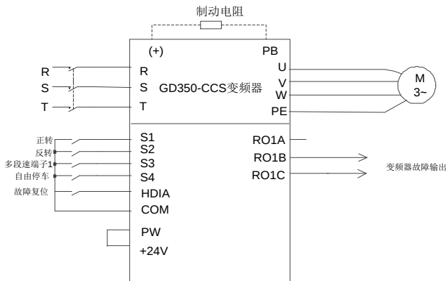
图 5-6 锥形电机接线参考
