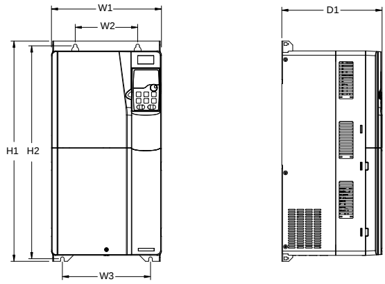
图 C-4 380V 45~75kW 壁挂安装
