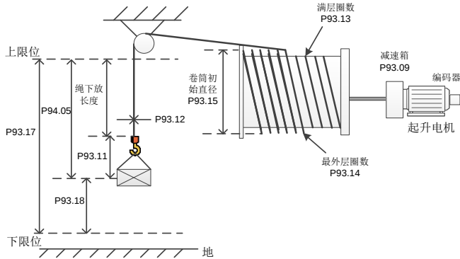
图 5-2 内部测量（电机编码器）：使用滑轮组
