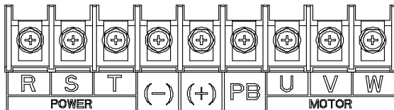
图 4-9 三相 380V 45~110kW 主回路端子
