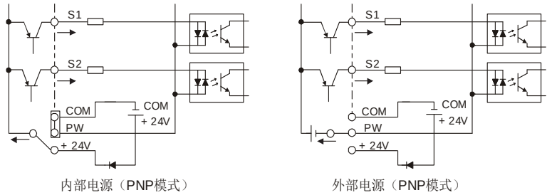
图 4-21 PNP 模式
