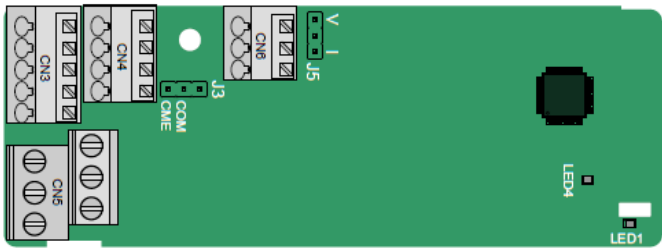
图 A-4 扩展卡地线连接
