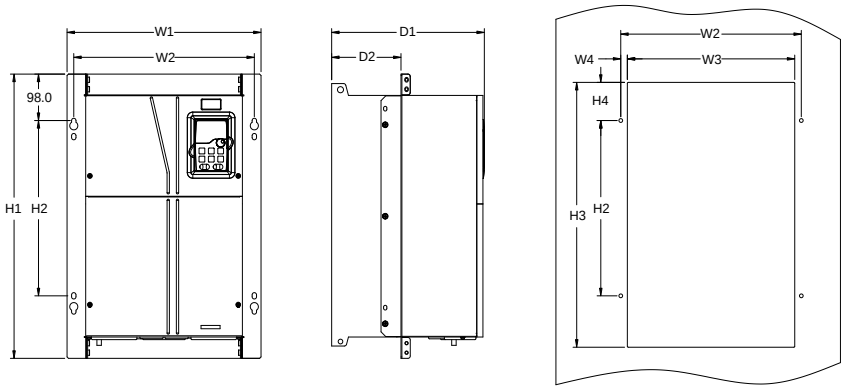
图 C-19 660V 22~132kW 法兰安装
