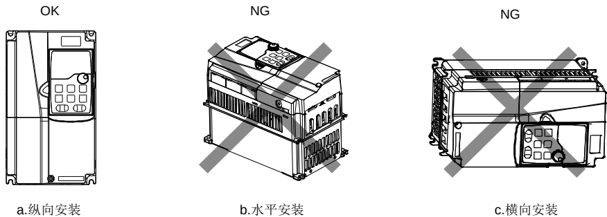
图 4-1 变频器安装方向
