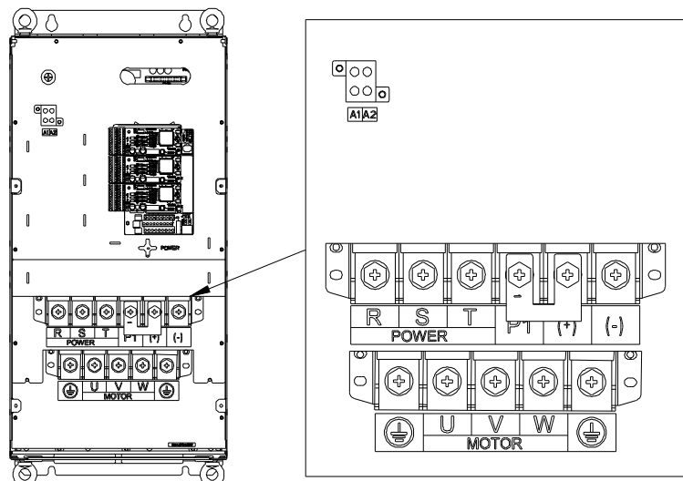
图 4-13 660V 55~132kW 主回路端子
