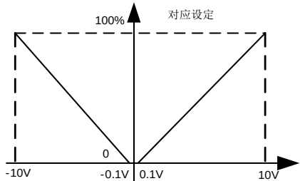
图 5-4 AI2 模拟量输入对应频率设定（选用模拟量给定选用-10V~10V）
