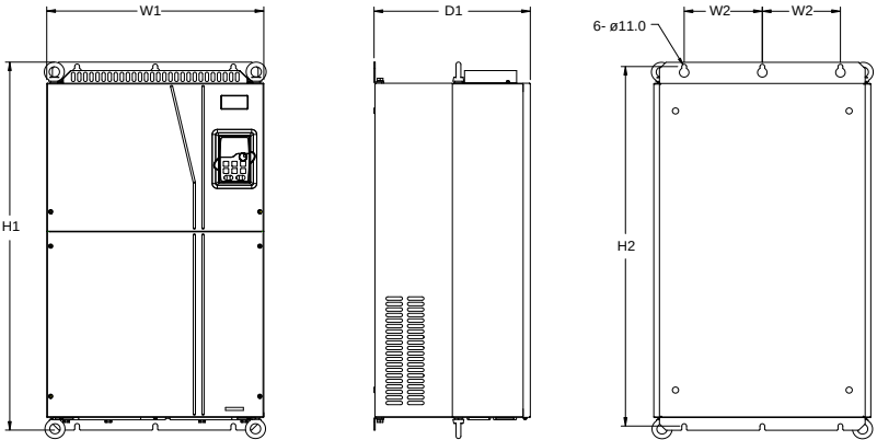
图 C-17 660V 160~220kW 壁挂安装
