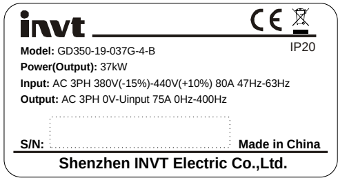
图 3-6 产品铭牌
