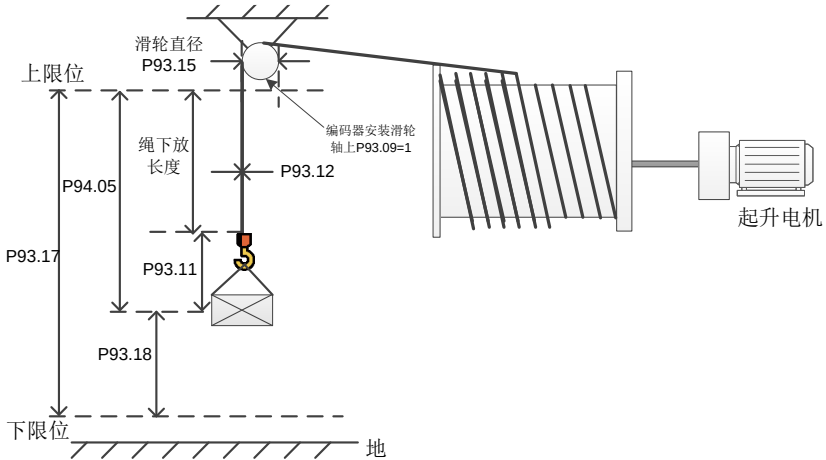
图 5-10 外部测量（HDI）
