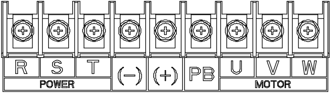
图 4-11 三相 380V 45~110kW 主回路端子
