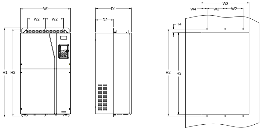
图 C-13 380V 132~200kW 法兰安装
