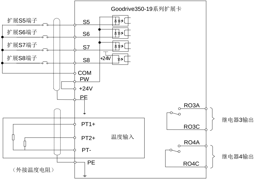
图 4-22 I/O 扩展卡 2 控制回路接线
