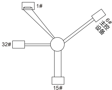
图 11-5 星形接法
