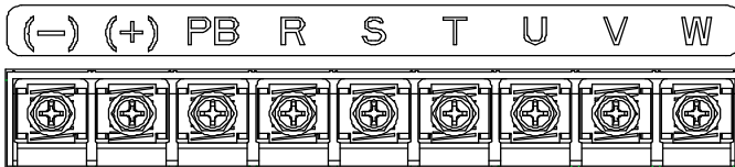
图 4-10 三相 380V 30~37kW 主回路端子
