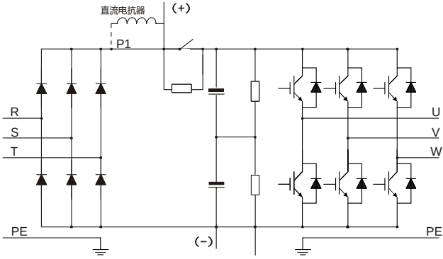
图 3-4 380V 132kW~315kW 主回路简图
