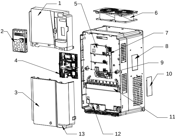
图 3-8 产品结构
