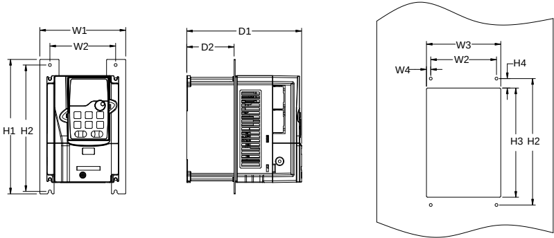
图 C-11 380V 1.5~75kW 法兰安装
