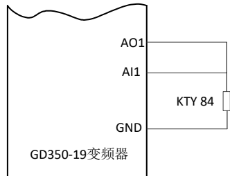
图 5-22 模拟量端口与 KTY84 接线
