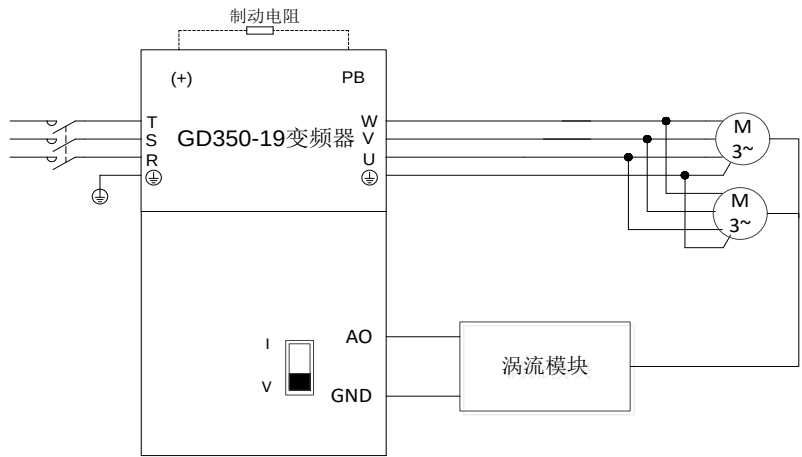
图 5-15 AO 端子和涡流模块接线
