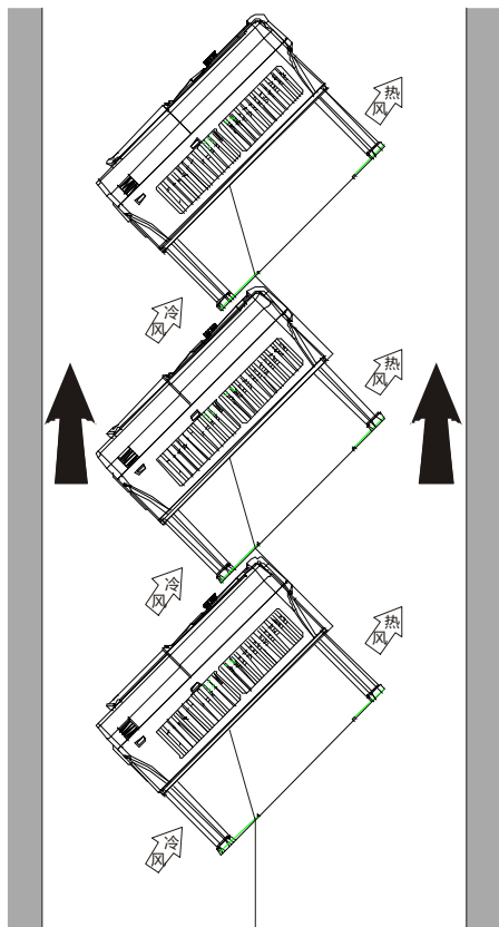
图 4-6 倾斜安装
