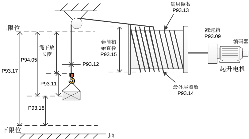
图 5-5 内部测量（电机编码器）：使用滑轮组
