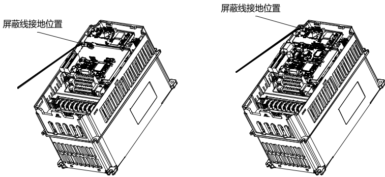
图 A-4 扩展卡地线连接
