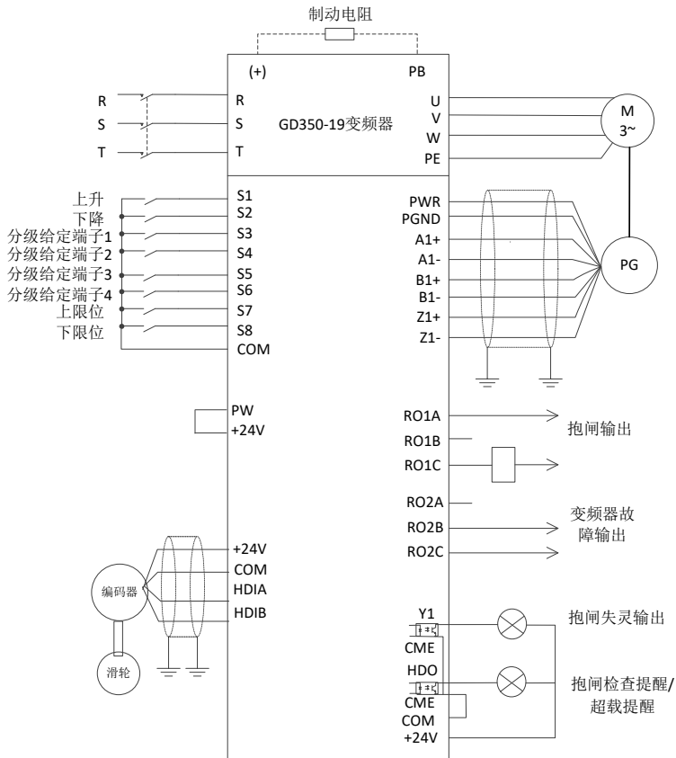
图 5-9 外部测量（HDI）接线（闭环）
