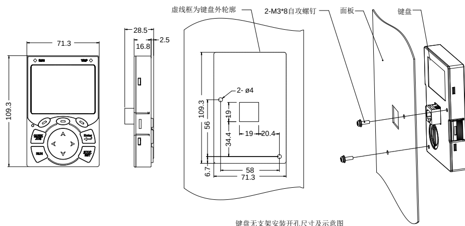
键盘无支架安装开孔尺寸及示意图
