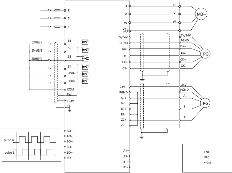
图 A-8 全闭环接 SSI 绝对式编码器和 24V 集电极开路信号增量式编码器
