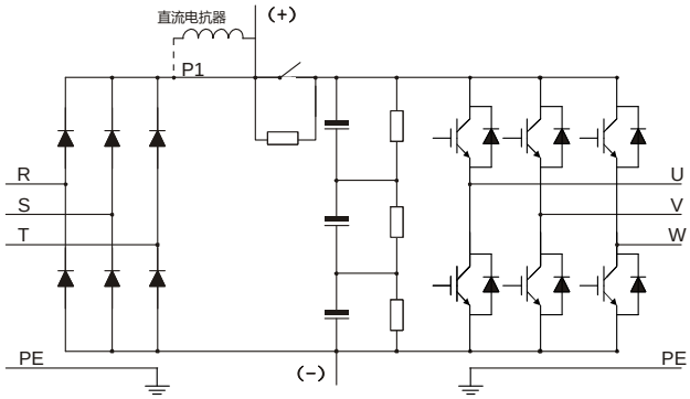
图 3-6 660V 全系列主回路简图
