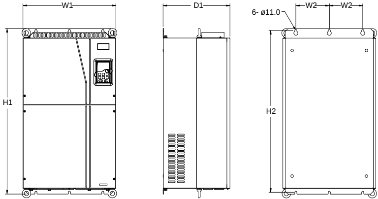
图 C-9 380V 132~200kW 壁挂安装
