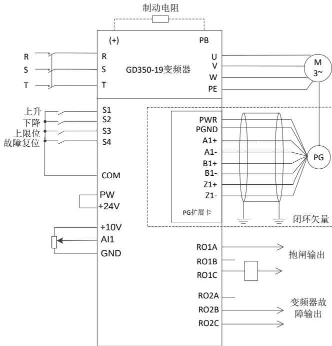
图 5-2 矿井、卷扬、绞车应用接线参考（推荐模拟量给定选用 0V~10V）
