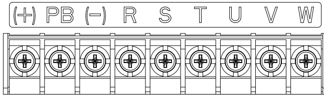
图 4-9 三相 380V 22kW（含）以下主回路端子
