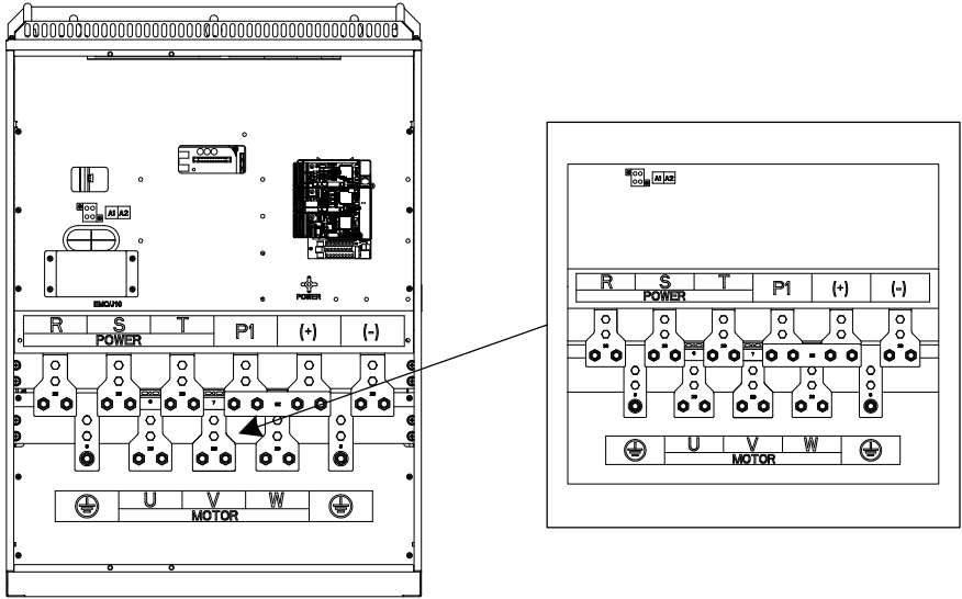
图 4-15 380V 220~315kW（无 A1、A2）、660V 250~355kW 主回路端子
