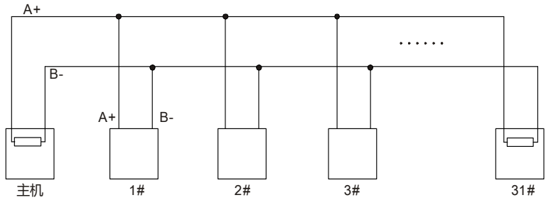
图 11-3 菊花简化接线
