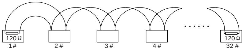
图 11-2 菊花接法现场接线
