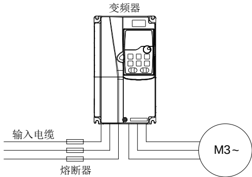
图 4-24 熔断器配置
