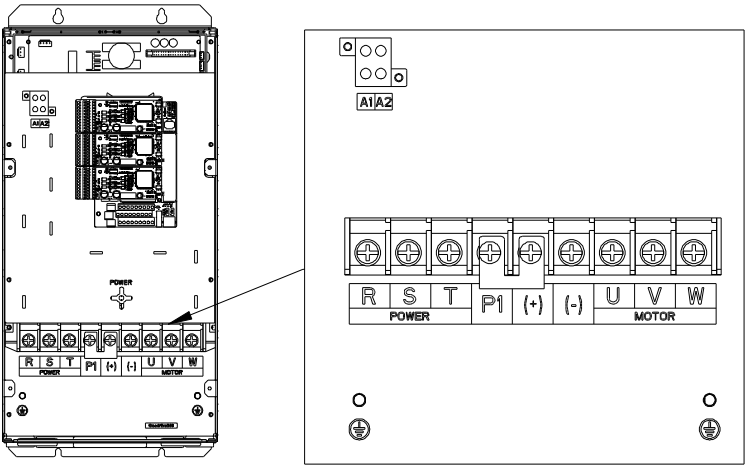
图 4-12 660V 22~45kW 主回路端子
