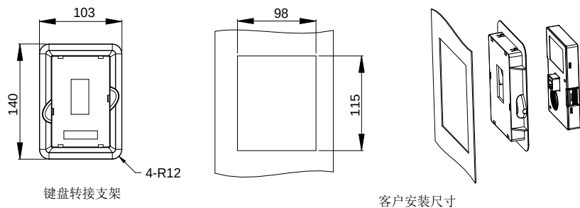
图 C-4 380V 1.5~500kW、660V 22~630kW 键盘安装架 (选配)
