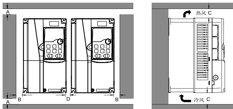
图 4-4 并行安装
