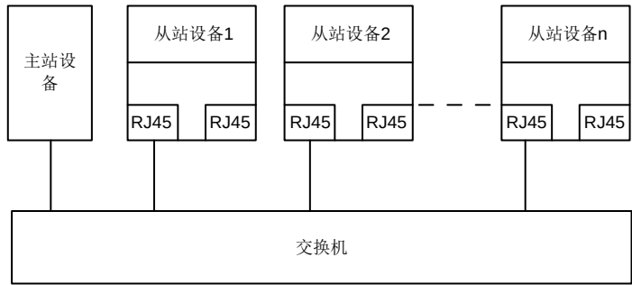
图 A-6 星型网络拓扑电气连接
