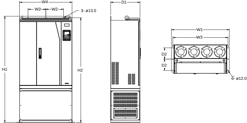
图 C-14 380V 220~315kW 落地安装
