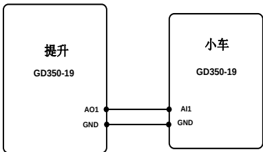
塔吊应用
