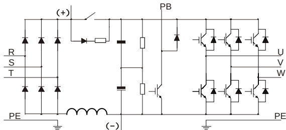
图 3-3 380V 30kW~75kW 主回路简图
