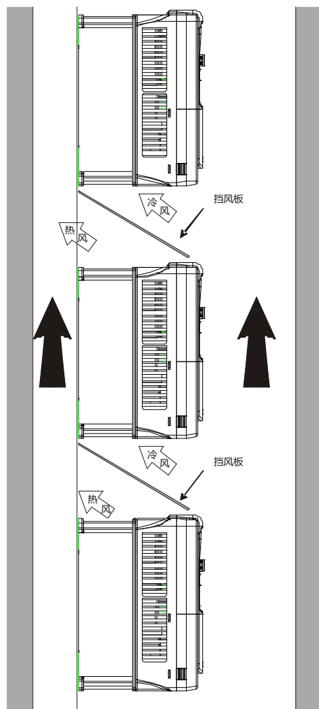
图 4-5 垂直安装
