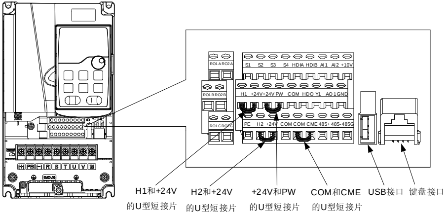
图 4-19 U 型短接位置
