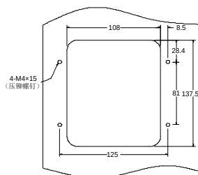
图 C-2 380V 37~315kW、660V 22~630kW 键盘安装架（标配）
