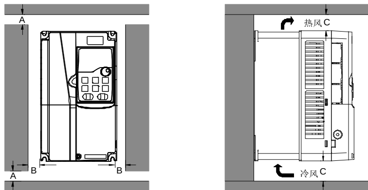
图 4-3 单台安装
