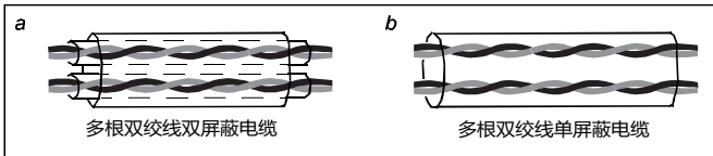
图 D-23 动力电缆布线
