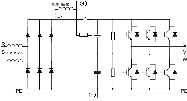
图 3-4 380V 132kW~315kW 主回路简图
