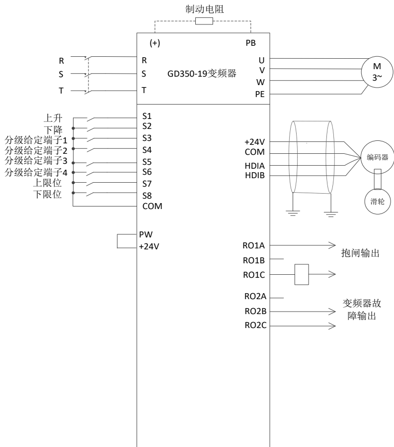
图 5-8 外部测量（HDI）接线（开环）
