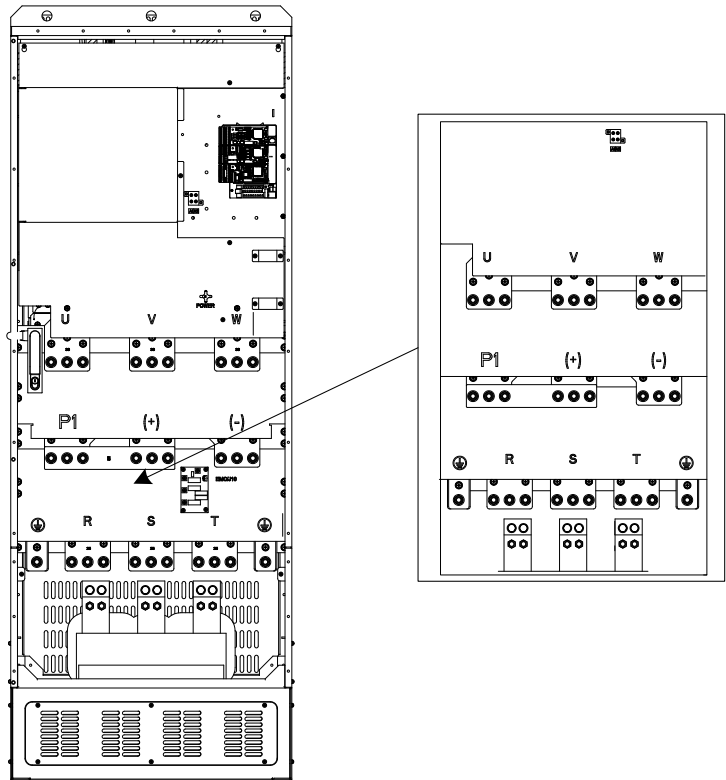
图 4-16 380V 355~500kW（无 A1、A2）、660V 400~630kW 主回路端子
