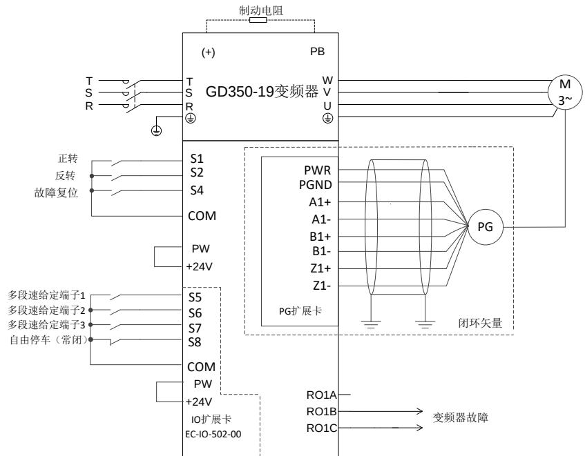
图 5-13 塔机回转应用接线
