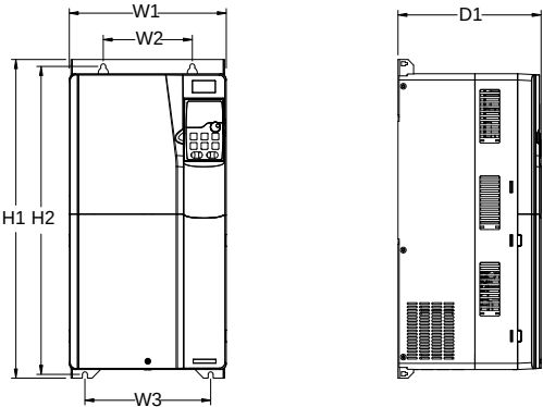
图 C-7 380V 45~75kW 壁挂安装
