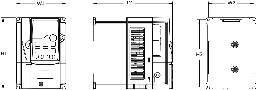
图 C-6 380V 1.5~37kW 壁挂安装
