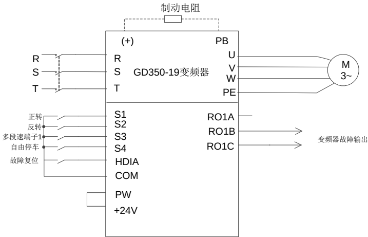
图 5-11 锥形电机接线参考
