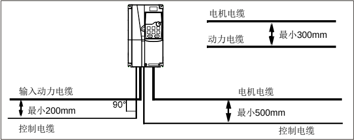
图 D-24 布线距离
