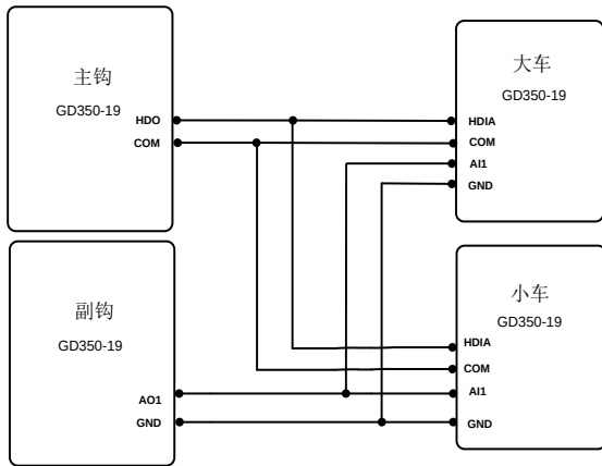
工厂/港口起重应用(双钩)
