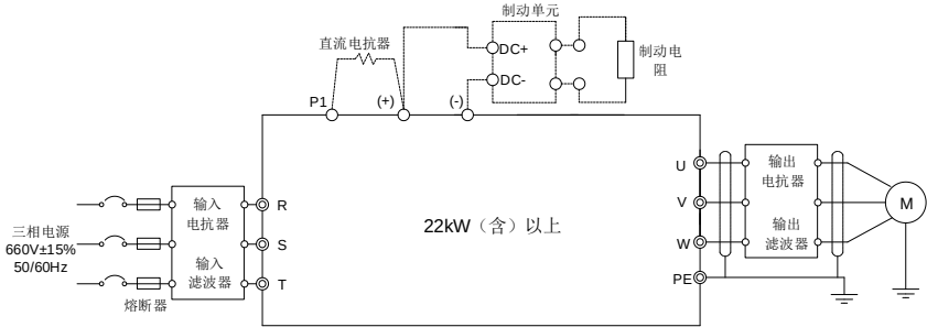
图 4-8 AC 3PH 520V(-15%)~690V(+10%)主回路接线
