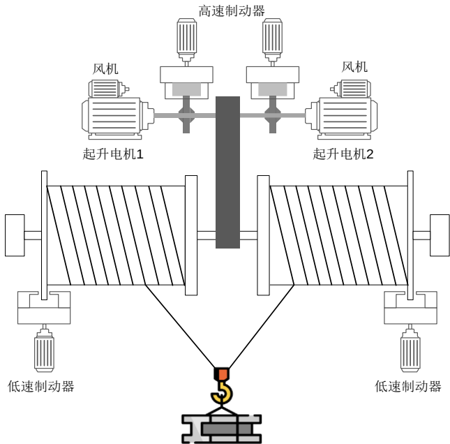
图 5-18 机械结构 1
