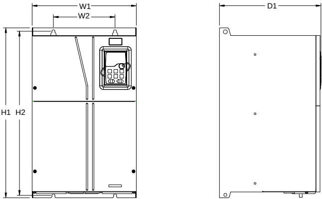
图 C-16 660V 22~132kW 壁挂安装
