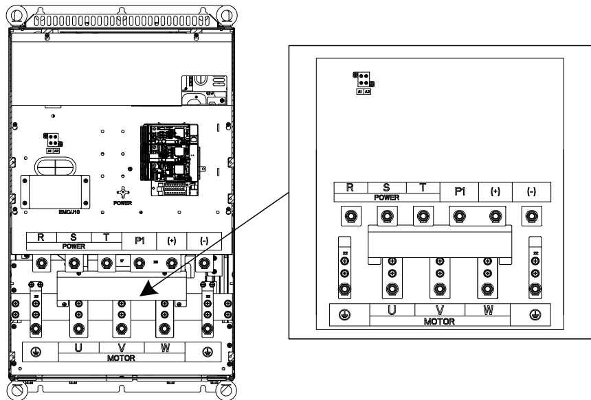
图 4-14 380V 132~200kW (无 A1、A2)、660V 160~220kW 主回路端子
