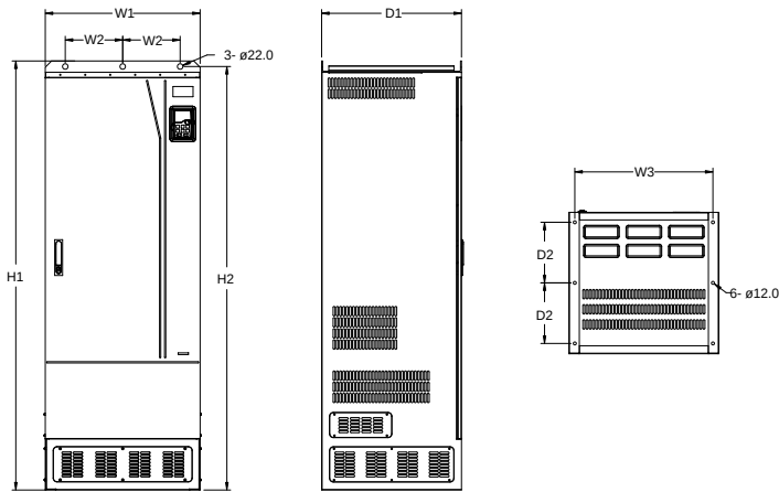
图 C-22 660V 400~630kW 落地安装
