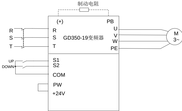
图 5-16 电动电位器调试接线
