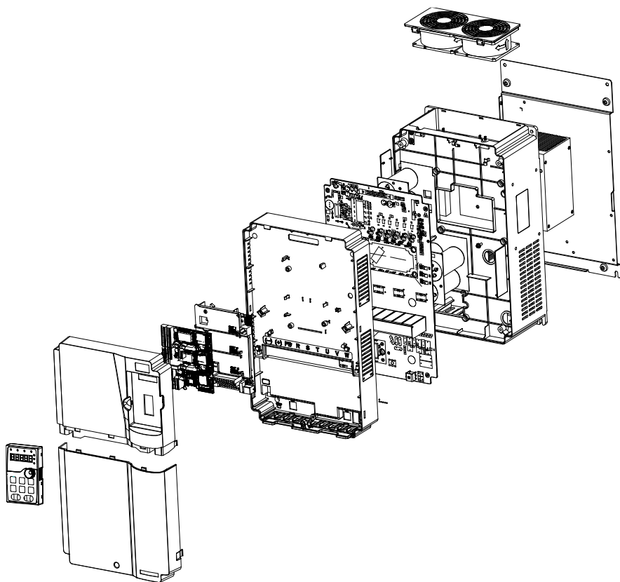
图 C-5 变频器结构
