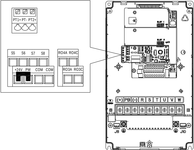
图 4-23 I/O 扩展卡 2 端子排列
