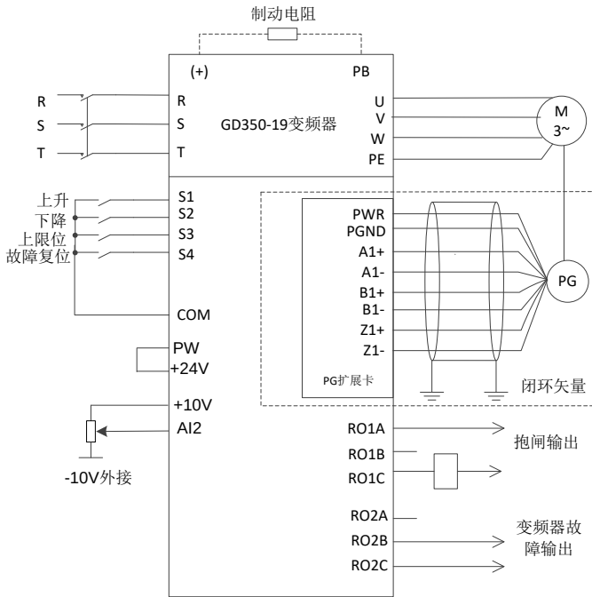
图 5-3 矿井、卷扬、绞车应用接线参考（模拟量给定选用-10V~10V）
