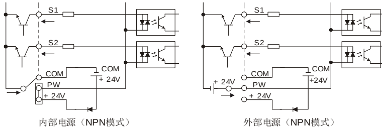
图 4-20 NPN 模式
