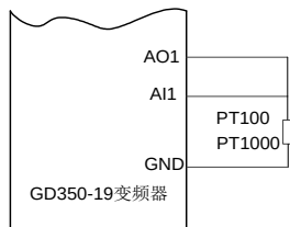
图 5-21 模拟量端口与 PT100/PT1000 接线
