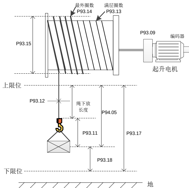
图 5-6 内部测量（电机编码器）：未使用滑轮组
