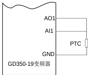
图 5-23 模拟量端口与 PTC 接线
