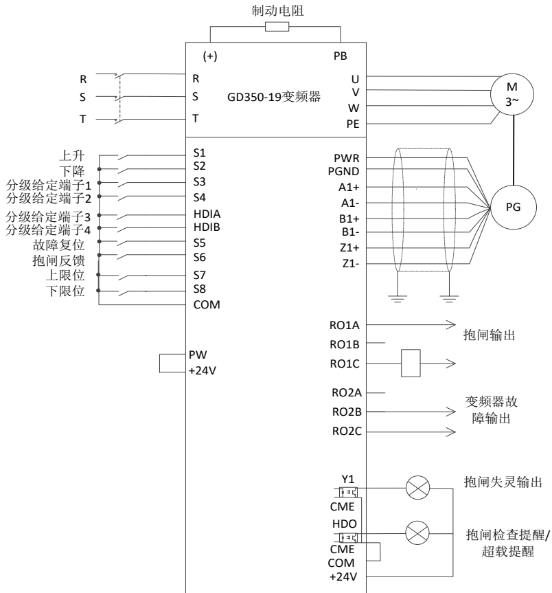
图 5-7 内部测量（电机编码器）接线
