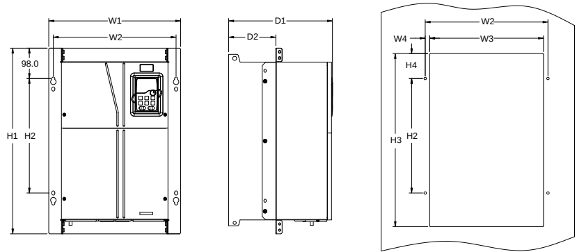
图 C-12 380V 90~110kW 法兰安装
