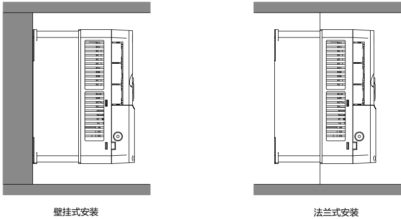
图 4-2 安装方式
