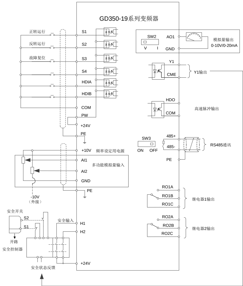
图 4-18 基本控制回路接线
