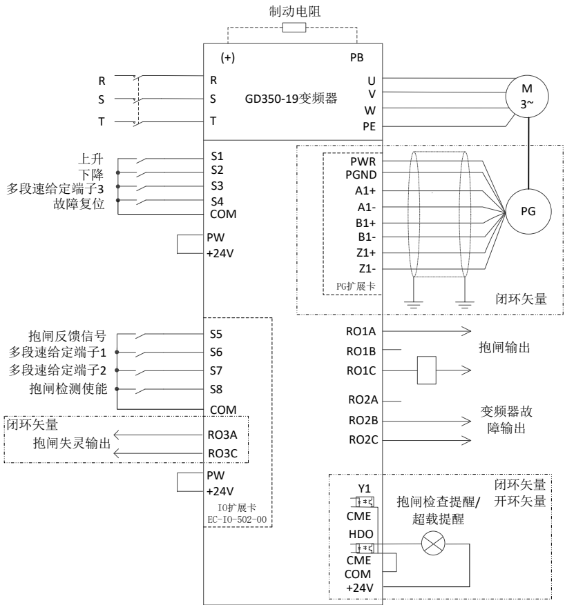
图 5-1 提升应用接线
