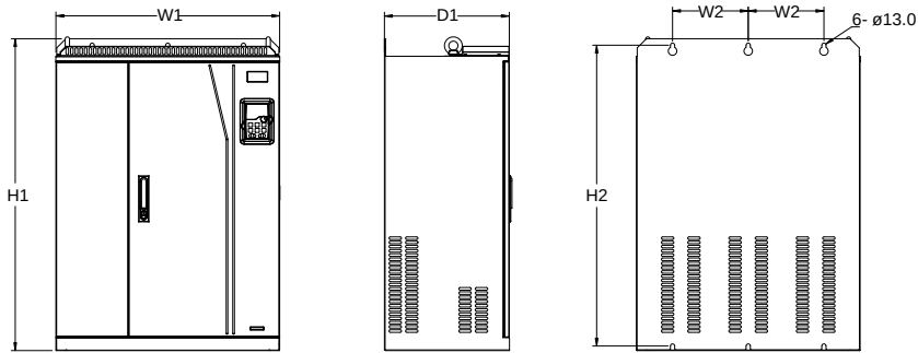
图 C-18 660V 250~355kW 壁挂安装
