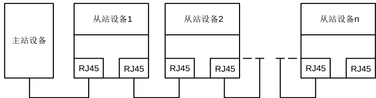
图 A-5 线型网络拓扑电气连接
