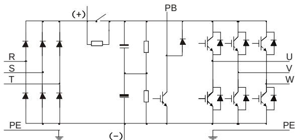
图 3-1 380V 15kW（含）以下主回路简图
