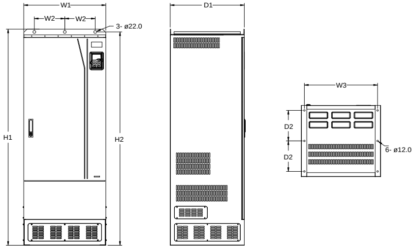
图 C-15 380V 355~500kW 落地安装
