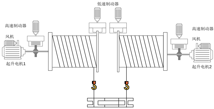
图 5-19 机械结构 2
