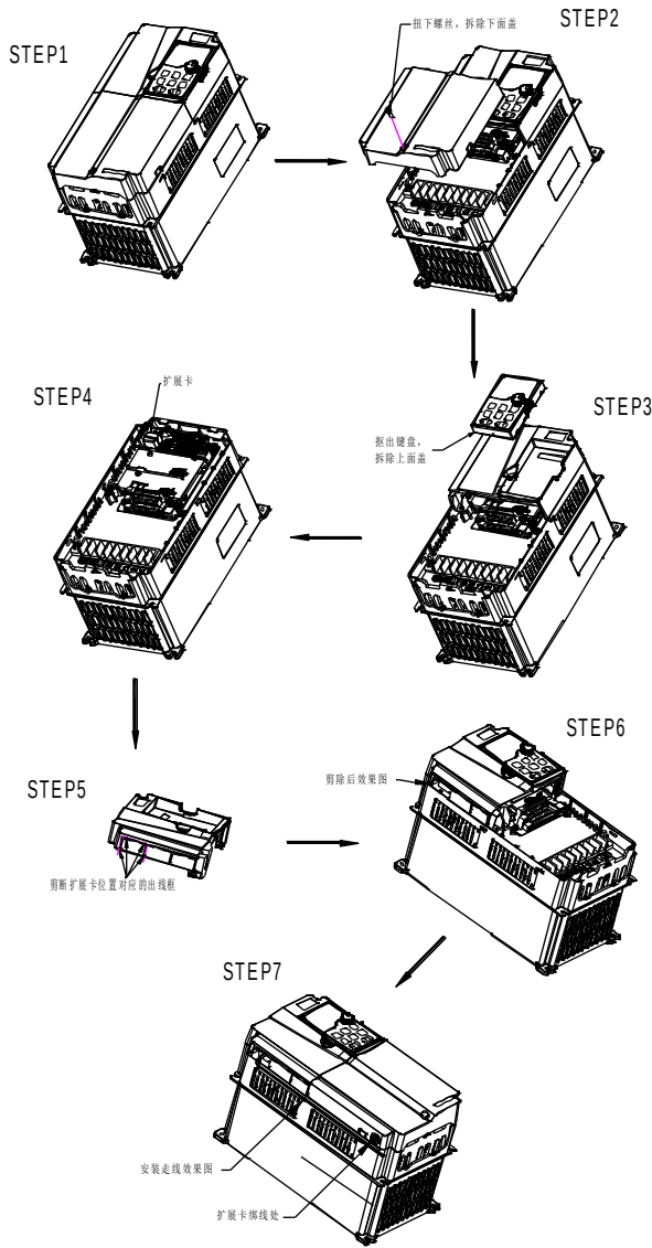
图 A-3 扩展卡安装步骤
