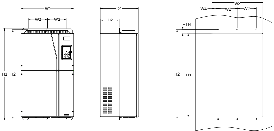
图 C-20 660V 160~220kW 法兰安装
