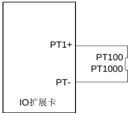
图 5-20 PT100/PT1000 使用扩展卡进行温度测量
