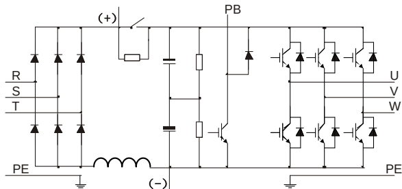
图 3-2 380V 18.5kW~22kW、90~110kW 主回路简图
