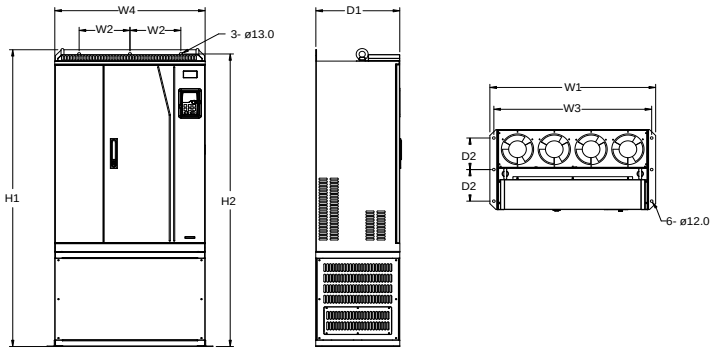
图 C-21 660V 250~355kW 落地安装
