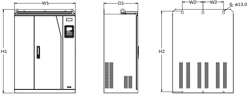
图 C-10 380V 220~315kW 壁挂安装
