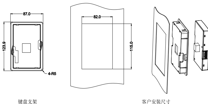
图 C-1 380V 1.5~315kW、660V 22~630kW 键盘安装架（选配）
